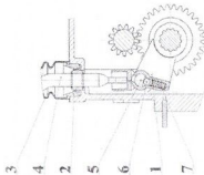
Рисунок 6 – Коробка переключения передач. Цеперечный разрез.
