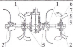
Рисунок 14а - Культиватор КМВ1.001.000.2.
