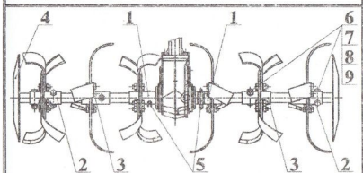
Рисунок 14г - Культиватор КМВ1.001.000.2-03.
