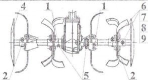
Рисунок 14б - Культиватор КМВ1.001.000.2-01.
