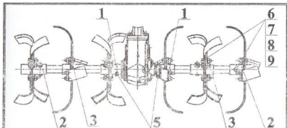
Рисунок 14в - Культиватор КМВ1.001.000.2-02.
