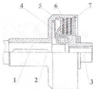
Рисунок 3 – Сцепление.
