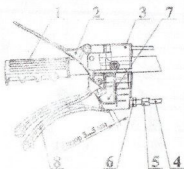
Рисунок 9 - Рукоятка руля левая.
