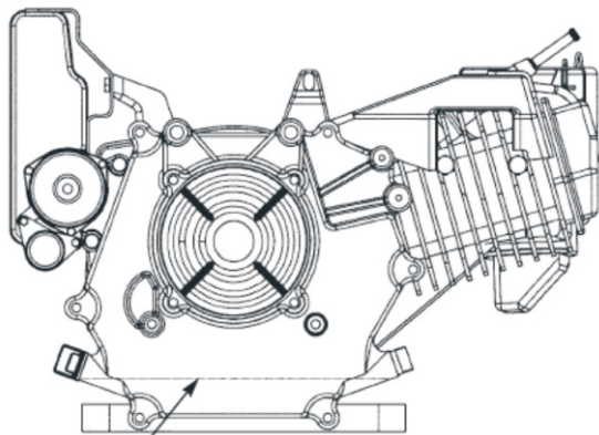
Уровень масла
