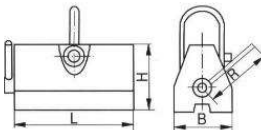
Рисунок 2. Габаритные размеры магнитного захвата
